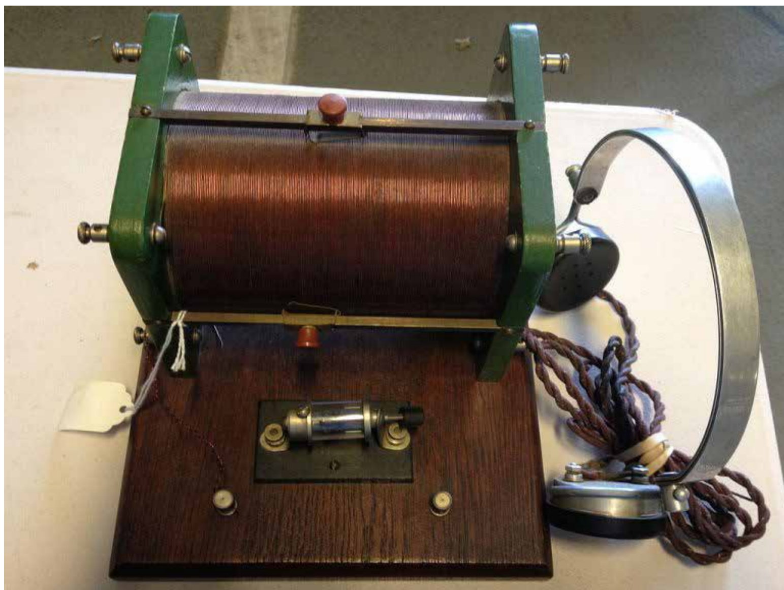
El primero en dar un paso fue el escocés James Clerk Maxwell, que presentó la Teoría Electromagnética en 1867, en la que, mediante cálculos matemáticos, predijo la posibilidad de crear ondas electromagnéticas y propagarlas por el espacio.
