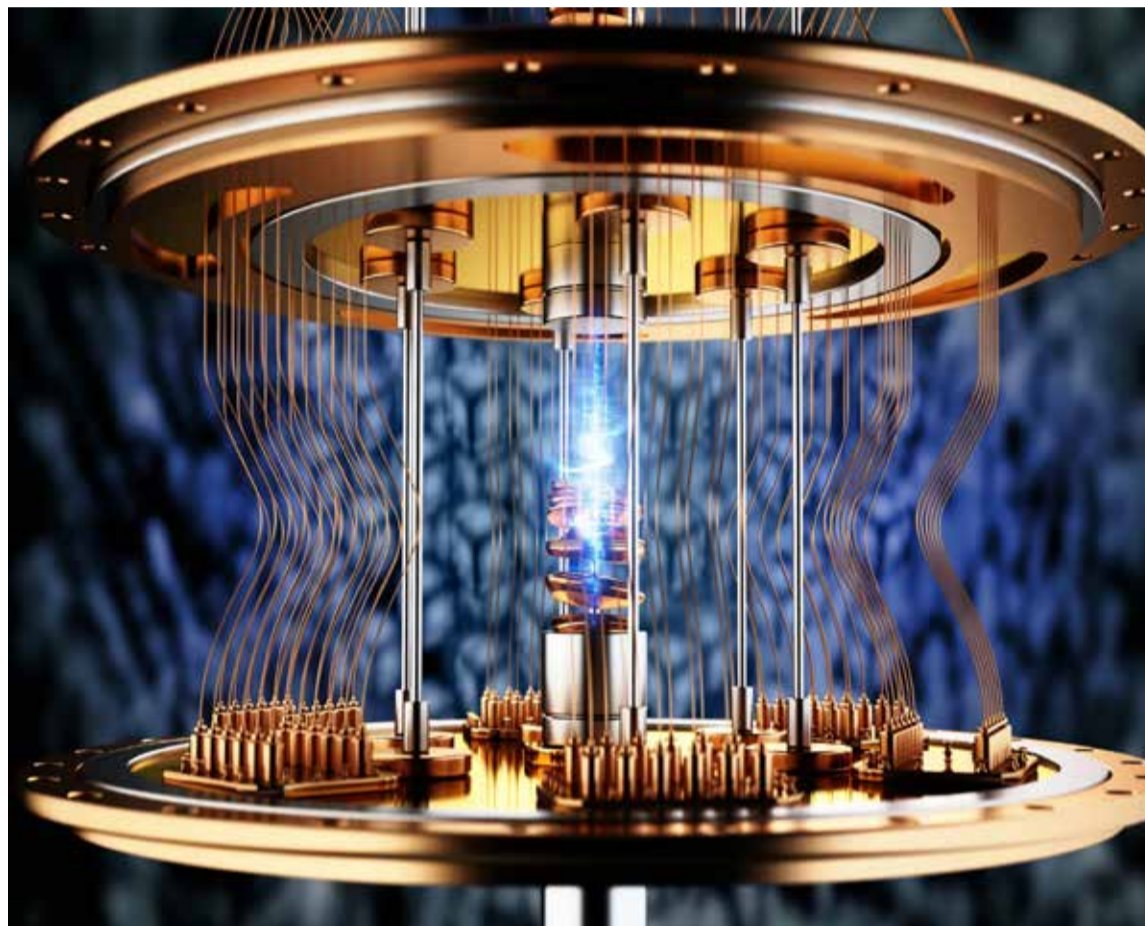
Computación Cuántica
